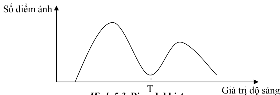
Hình 5.3. Bimodal histogram
